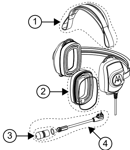
Figura 5: Piezas de repuesto, PMLN8085
