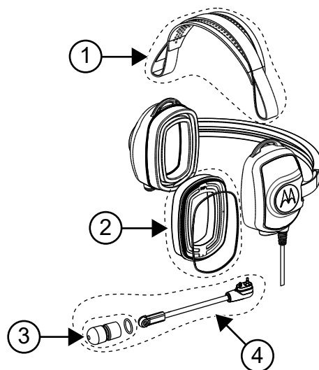
Figura 5: Peças de reposição do PMLN8085
