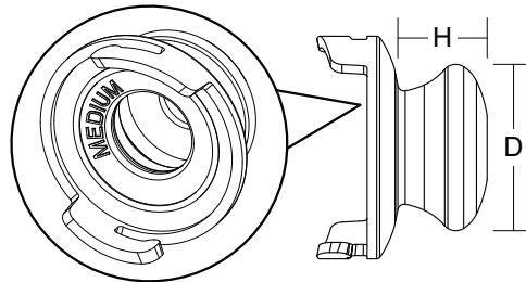
Figure 8 : Taille et mesure des embouts
