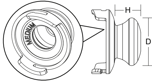
Рисунок 8 . Розмір вкладиша та габарити
