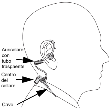
Figura 2: Collegamento dell'accessorio
