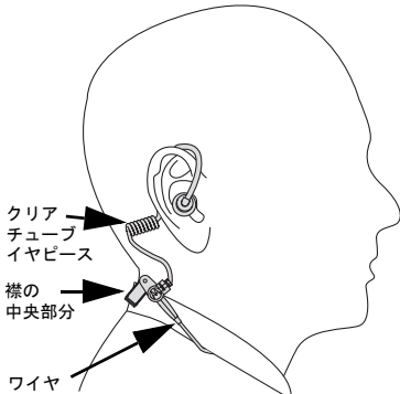
図 2: 本アクセサリの装着
