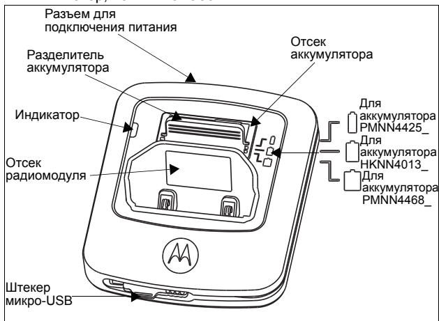
Рис. 1: Зарядное устройство, рассчитанное на три устройства
