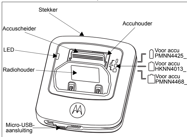
Figuur 1: Tri-Unit-oplader
