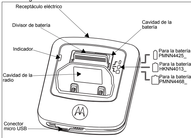
Figure 1: Cargador de tres unidades
