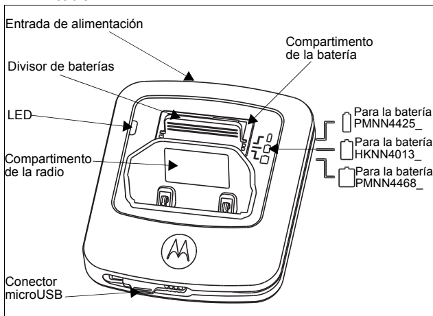
Figura 1: Cargador triple
