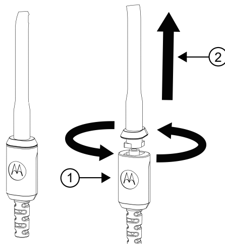
Figura 6: Substituição do tubo acústico translúcido
