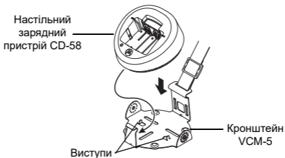
Рис. 3: Установлення настільного зарядного пристрою CD-58 у кронштейн VCM-5
