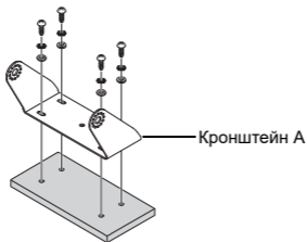
Рис. 1: Установлення кронштейна А
