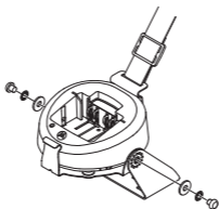
Рис. 5: Установлення кронштейна VCM-5 на кронштейні А
