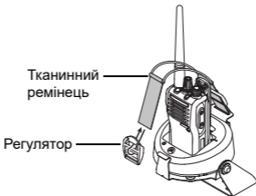
Рис. 8: Установлення регулятора в тканинний ремінець
