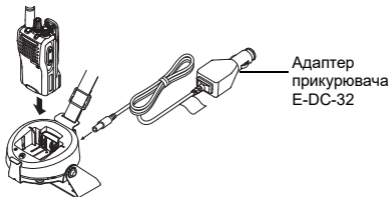
Рис. 7: Підключення адаптера прикурювача E-DC-32 до настільного зарядного пристрою CD-58
