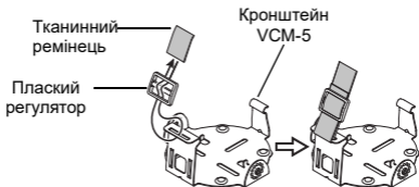
Рис. 2: Установлення тканинного ременя та плоского регулятора
