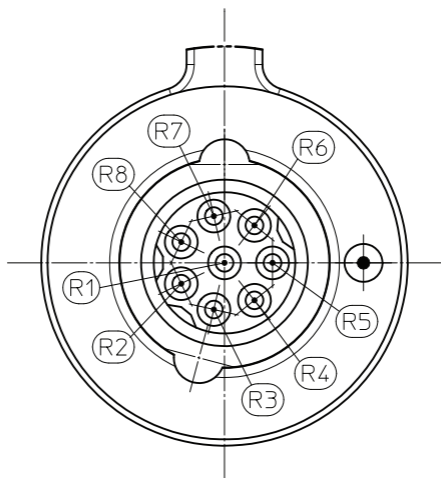
Abb. 3. Molex-Anschlussstiftbelegung
