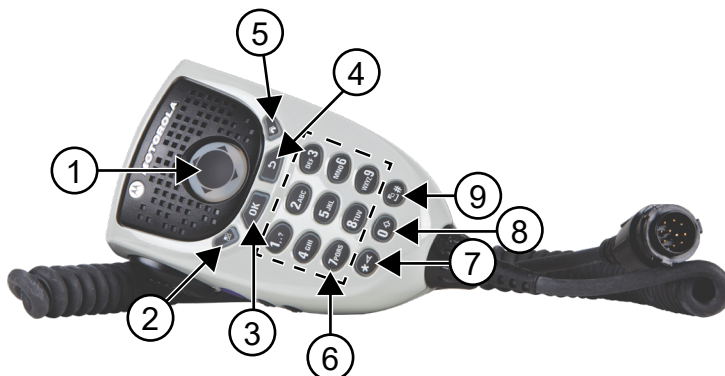
Рис. 5. Микрофон с клавиатурой IMPRES RMN5127_
