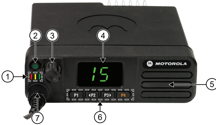
Şekil 4: Sayısal Ekranlı Model
