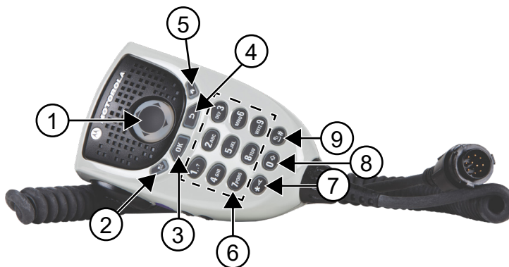
Rysunek 5: Mikrofon z klawiaturą IMPRES RMN5127_
