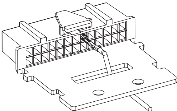
Figura 1a Protetor contra torção do fio
