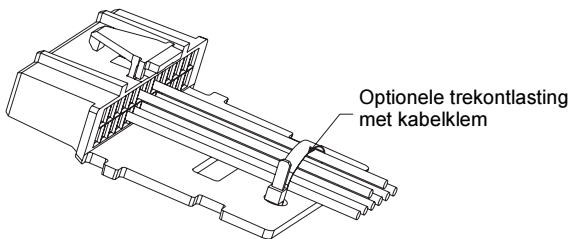
Afbeelding 1b. Optionele trekontlasting
