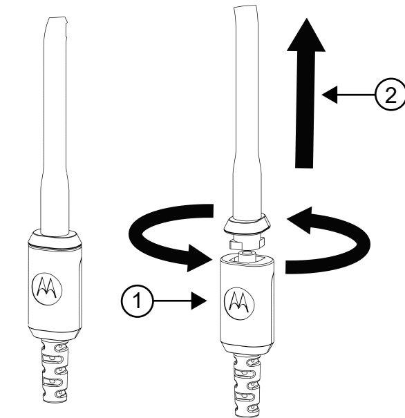
Figure 10 : Remplacement du tube acoustique transparent
