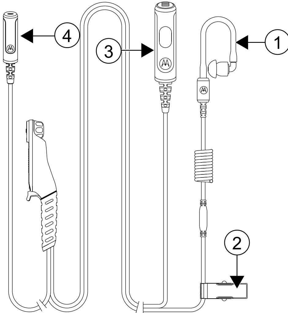
그림 1 : 이어폰 개요
