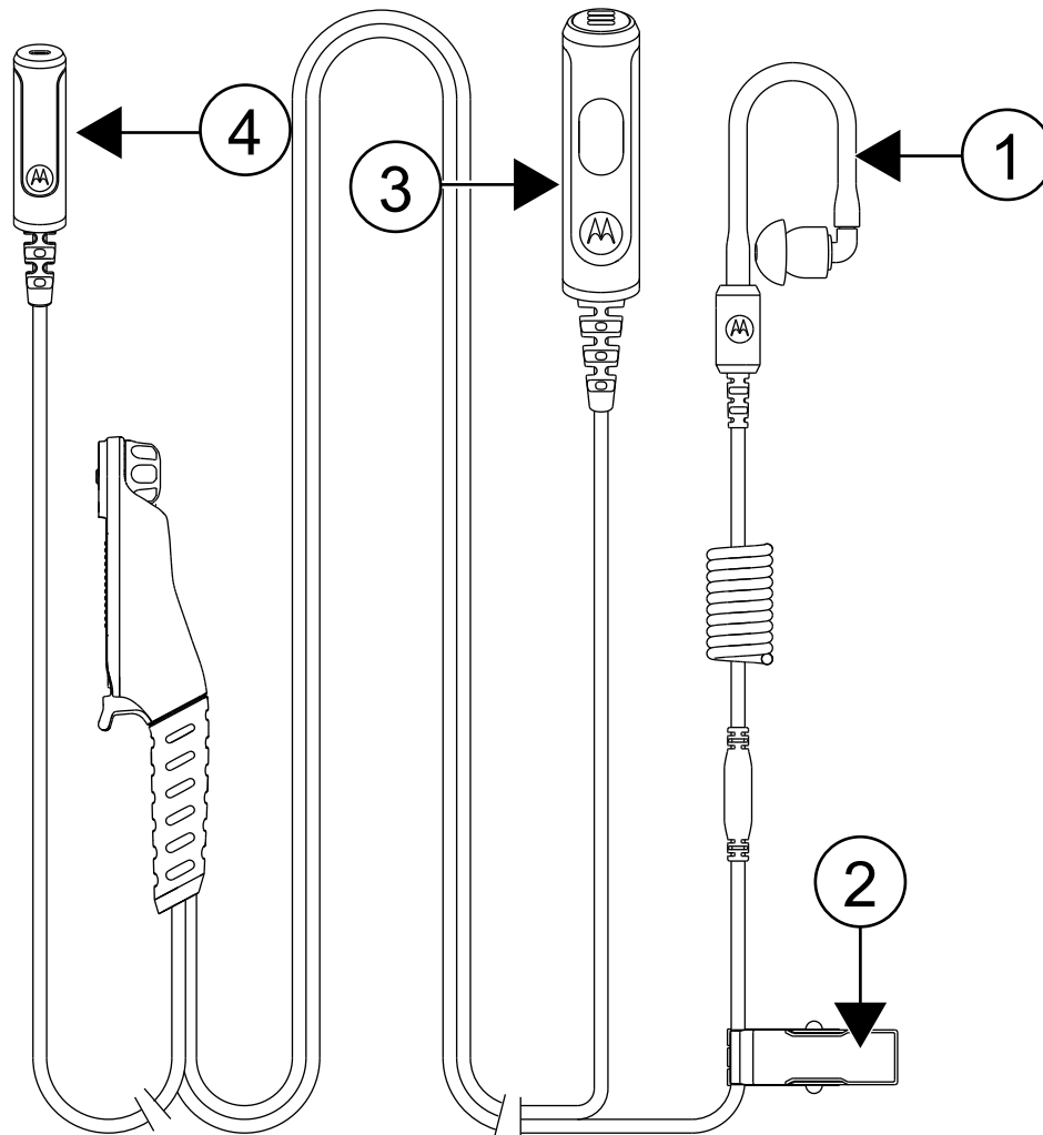
Рисунок 1 . Огляд навушника
