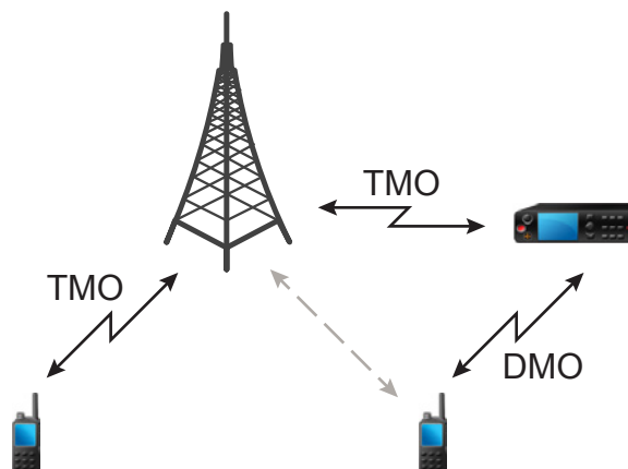
Figura 7 : Comunicación a través de puertas de enlace
