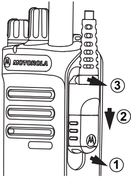
그림 5: 액세서리 커넥터를 키패드 미장착 무전기에 부착
