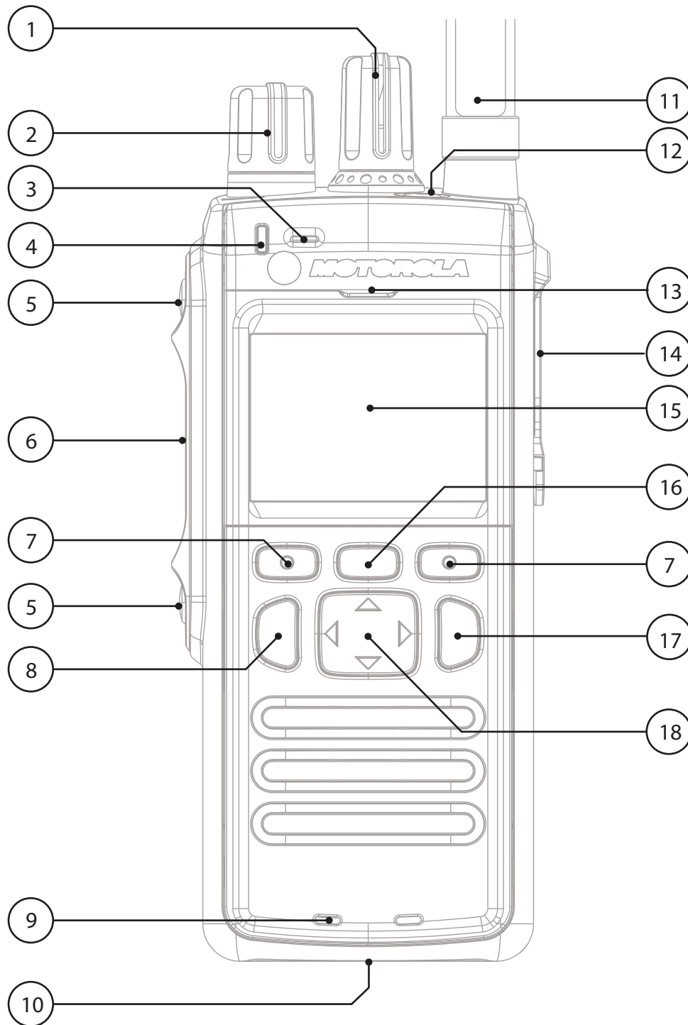
Acima 4 :Controles e indicadores da série MTP3x00
