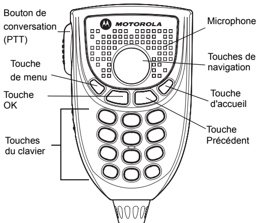
Microphone à clavier – vue avant
