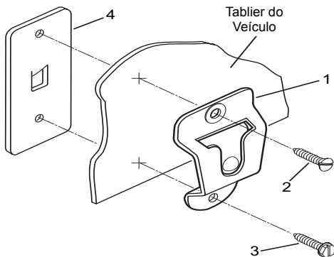
Clipe para Pendurar Microfone HLN9073
