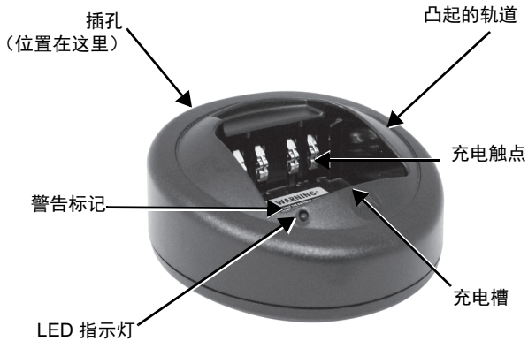
图 1: 电池充电器
