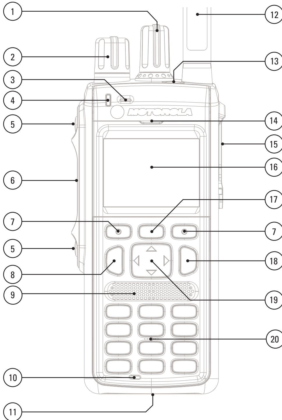
Figura 2 : Controles e indicadores da série MTP3x50
