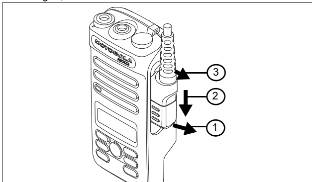
Abbildung 2: Entfernen Sie den Zubehörschlüssel
