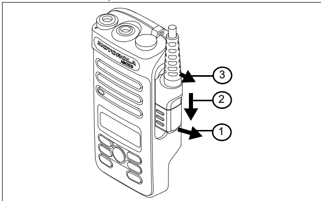
Figura 2: Rimozione del connettore accessori
