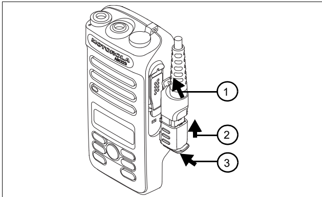
Figura 1: Fixe o conector do acessório
