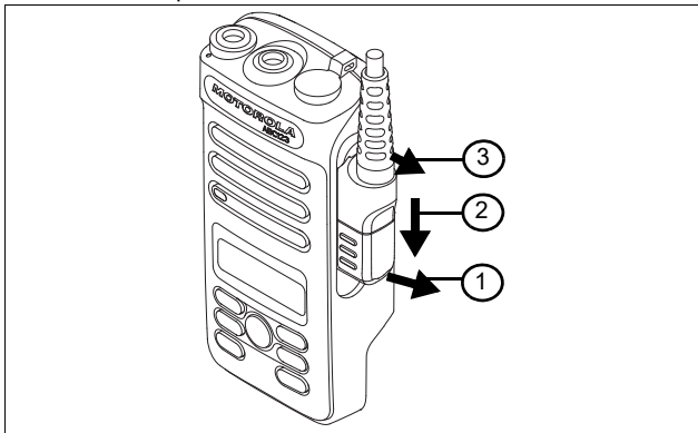
Figura 2: Remova o conector acessório
