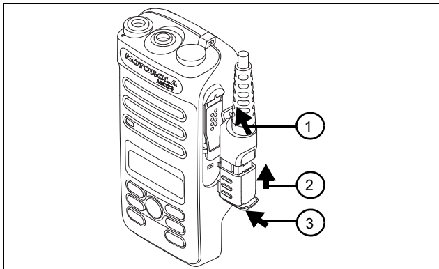
Figura 1: Fissaggio del connettore accessori
