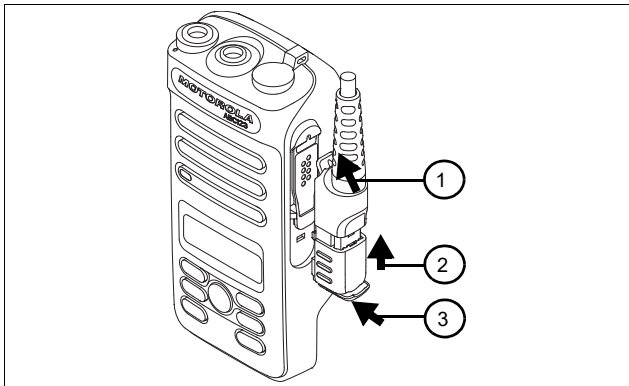
Рис. 1. Установка разъема для аксессуаров
