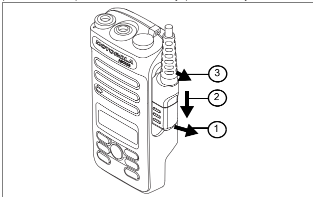
Рис. 2. Извлечение разъем для аксессуаров.
