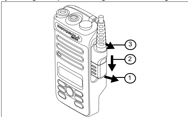
Afbeelding 2: De accessoireaansluiting verwijderen
