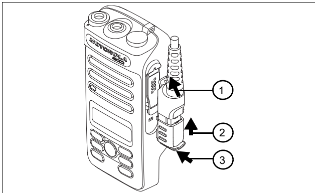
Afbeelding 1: De accessoireaansluiting bevestigen
