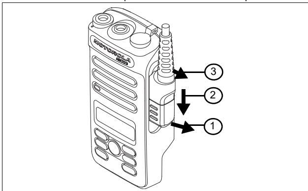
Figure 2 : Retrait du connecteur pour accessoires
