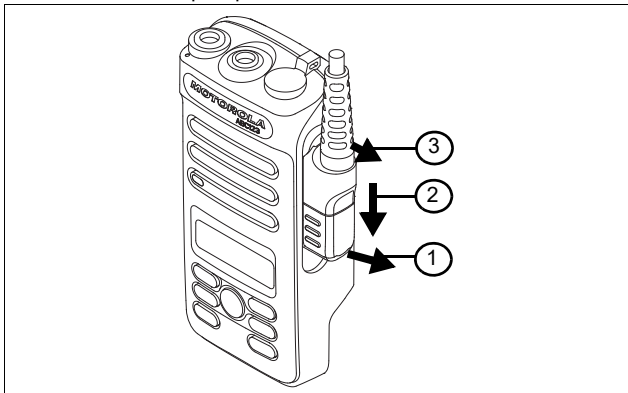
Figura 2: remova o conector do acessório
