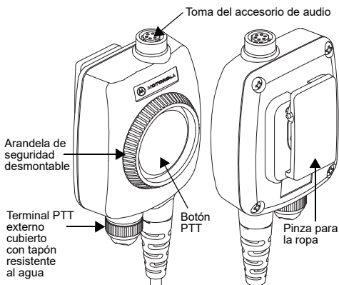
Figure 1. Descripción general del módulo de la interfaz
