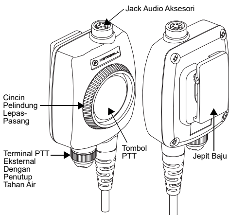
Gambar 1. Gambaran Umum Modul Antarmuka
