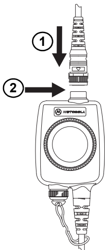
Afbeelding 2. Audioaccessoire bevestigen
