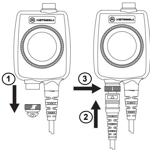
Gambar 3. Memasang PTT Jarak Jauh
