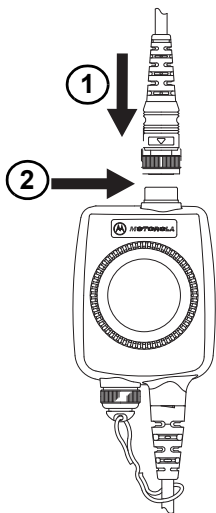
Рис. 2. Подключение аудиоаксессуаров
