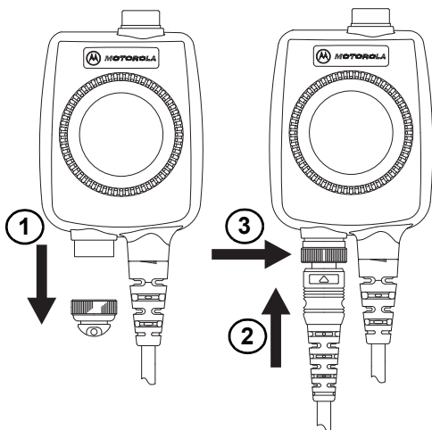
Figura 3. Fixar o PTT remoto
