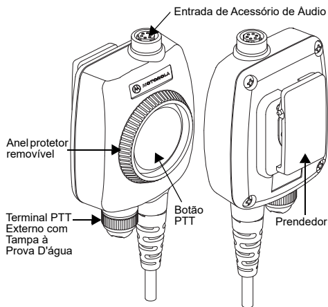
Figura 1. Visão geral de Módulo de Interface
