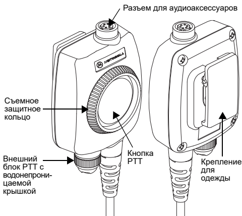
Рис. 1. Обзор интерфейсного модуля
