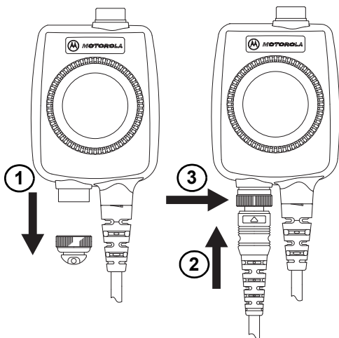
Рис. 3. Подключение кнопки удаленной связи РТТ
