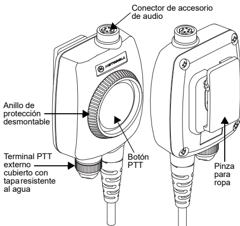
Figura 1. Descripción general del módulo de interfaz
