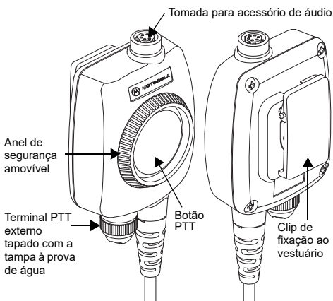
Figura 1. Descrição geral do Módulo de interface
