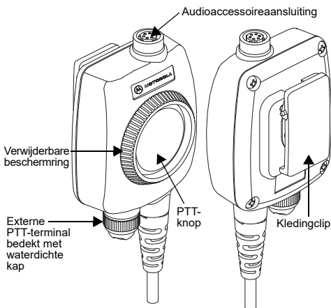
Afbeelding 1. Overzicht van de interfacemodule
