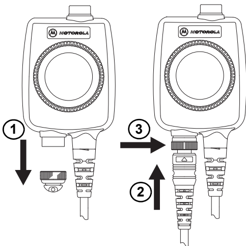
图 3. 安装远程 PTT 键
