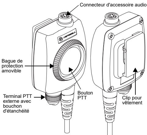
Figure 1. Vue d'ensemble du module d'interface
