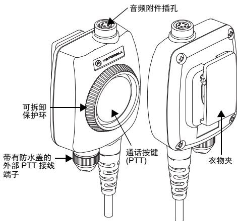
图 1.接口模块概述
