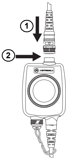
Figure 2. Conexión del accesorio de audio
