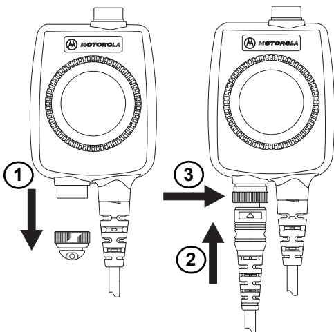
Abbildung 3. Anschließen der Remote-PTT
