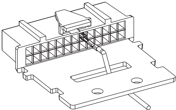
Figura 1a. Alívio de Tensão do Fio
