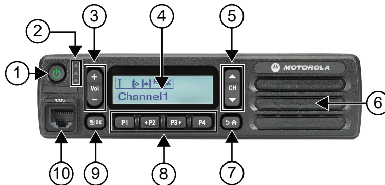
Figura 2: Modello con display alfanumerico
