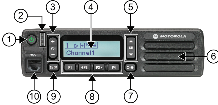
Şekil 2: Alfaisayisal Ekranlı Model
