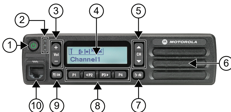
Abbildung 2: Modell mit alphanumerischem Display
